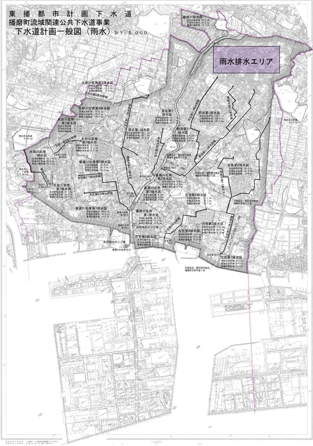
下水道計画一般図（雨水）
