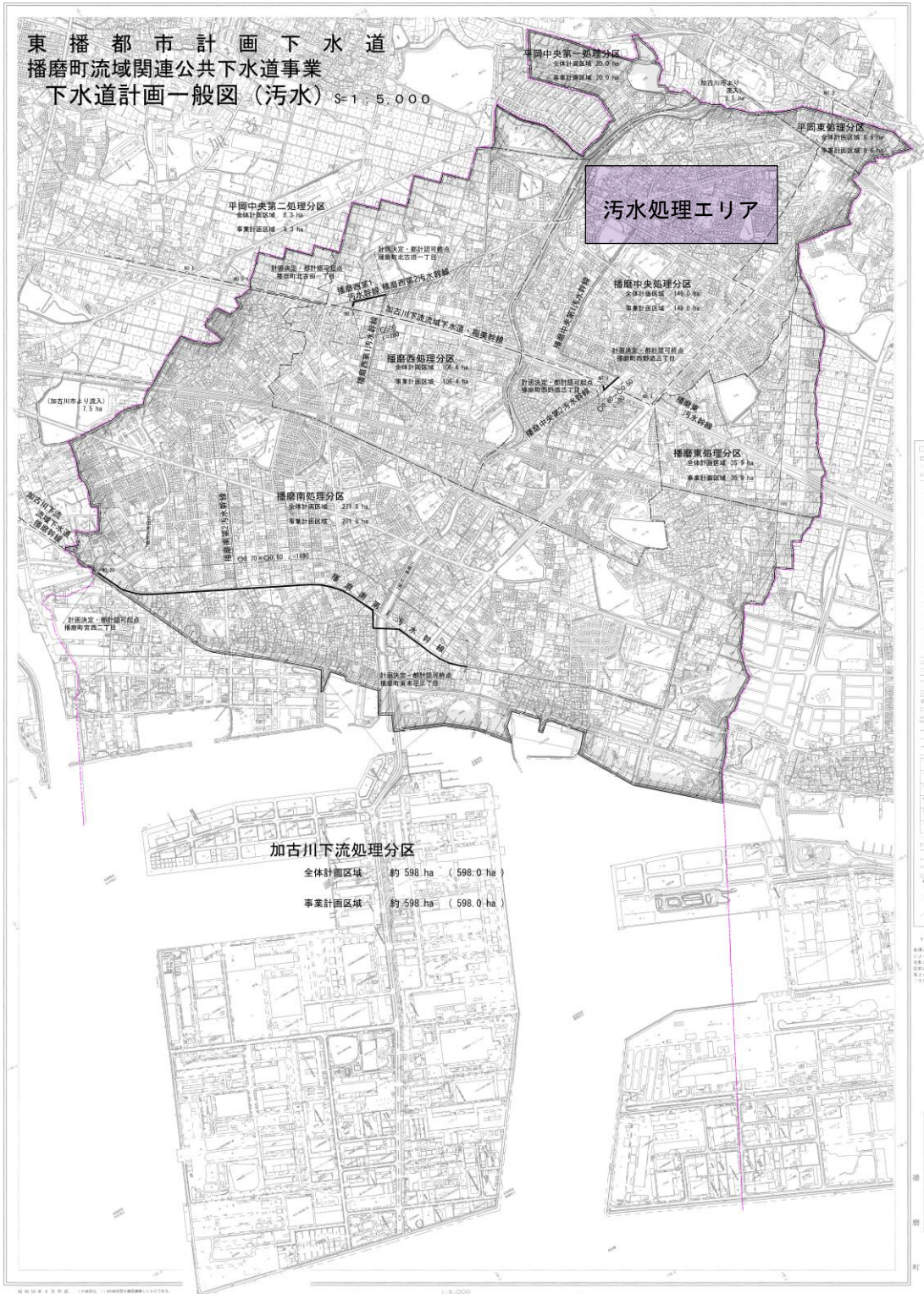
下水道計画一般図(污水)
