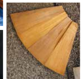
▲檜皮の切り方と、葺く際の重ね方で屋根の曲線を醸し出す
